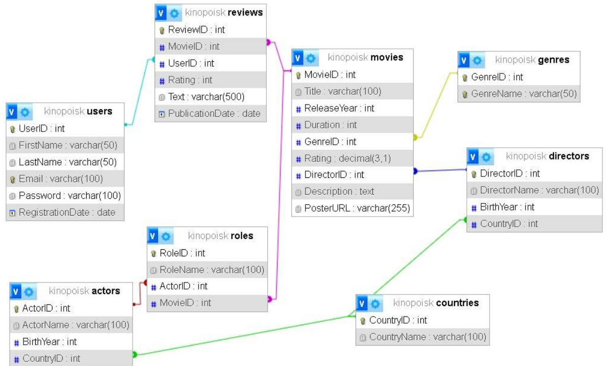
Рисунок 2 — EER-диаграмма базы данных
